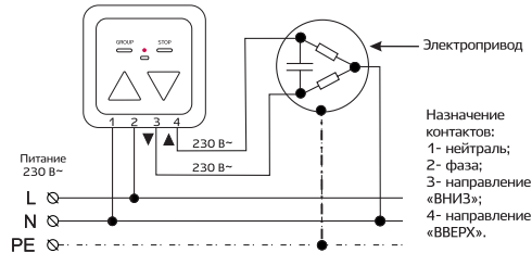
Рис. 3 — Подключение к сети и электроприводу
